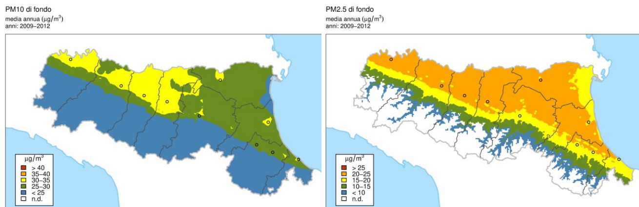
Figura 2. Stima della distribuzione del particolato ( PM_{10} e PM_{2,5} ) calcolata sul periodo 2009-2012
